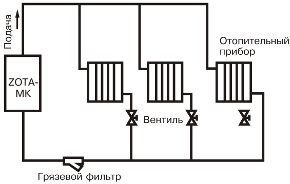
Рис.5 Упрощенная схема подключения микрокотельной в отопительную систему.
