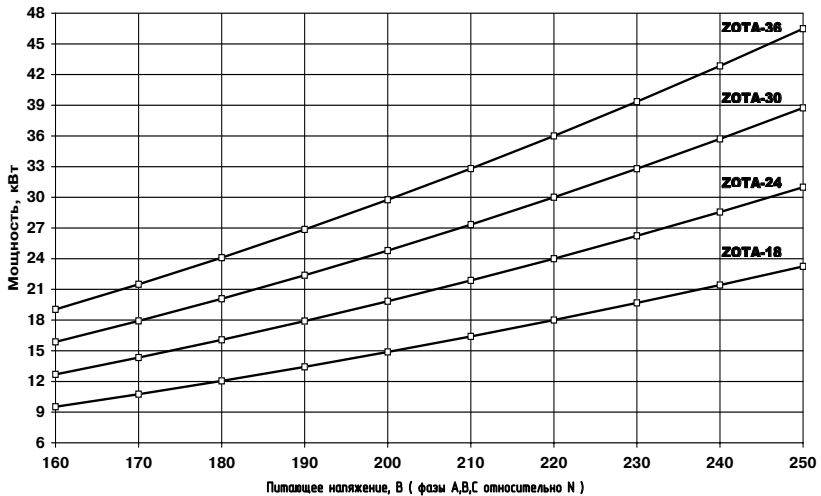
Рис.6 График изменения мощности микрокотельной в зависимости от питающего напряжения
